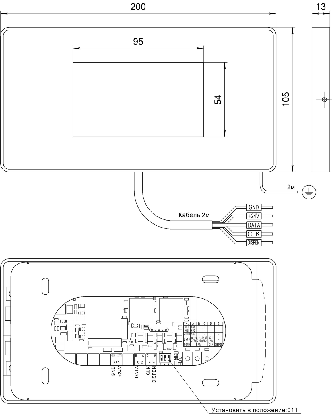
Рис.1 Внешний вид Табло накладное МАЛАХИТ НШЕК.468232.127-02 SIGMA (дисплей 4,3)
